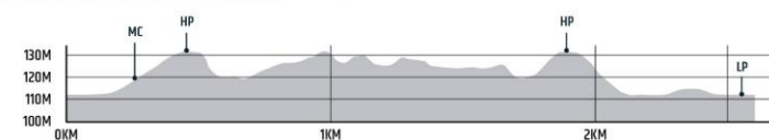
HÖJDPROFIL 2580m
